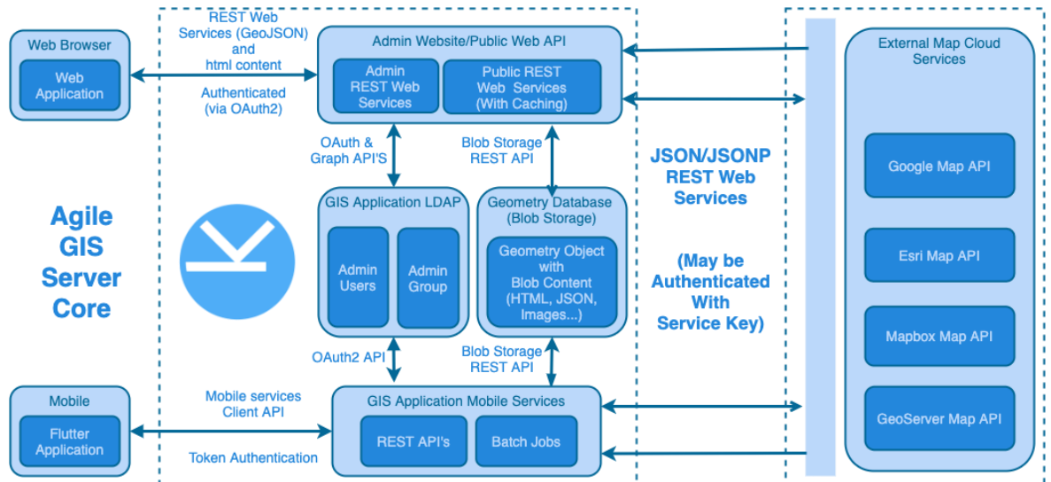
Hình 7.3 : Kiến trúc Gis Server Core
